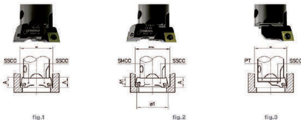
Fig. 1 – Na utilização de duas cápsulas SSCC usando juntas, ajustadas na mesma distância radial para operações de desbaste de alta velocidade. Fig. 2 – Na utilização de duas cápsulas diferentes, por exemplo uma SSCC e outra SMCC interpolando a usinagem, com distâncias radiais diferentes para operações de desbaste profundas. Fig. 3 – Os cabeçotes de mandrilhamento são ajustados com a possibilidade de utilizar somente uma cápsula, para operações de desbaste e acabamento com remoção leve de material. A placa de proteção para o serrilhado deve sempre ser usada para este tipo de operação.
