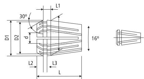
ER11 - ER50
