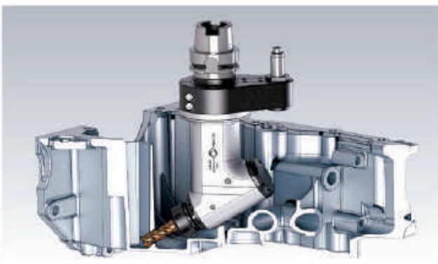
Cabeçote fixo com ângulo variável
